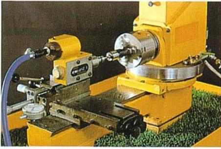
5番軸による内研専用機 Internal grinding with No. 5 Spindle
