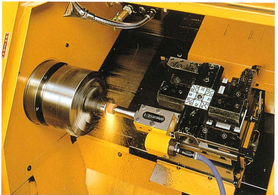
NC旋盤に取付けたGU-1によるワンチャック精密研磨 Mounted GU-1 on N/C Lathe for one chuck precise grinding
