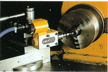
ダイヤモンド砥石による超硬テーパー穴研磨 Tapered hole grinding of carbide steel with vitrified diamond wheel
