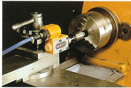
2番軸による内面研磨 Internal grinding with No. 2 Spindle
